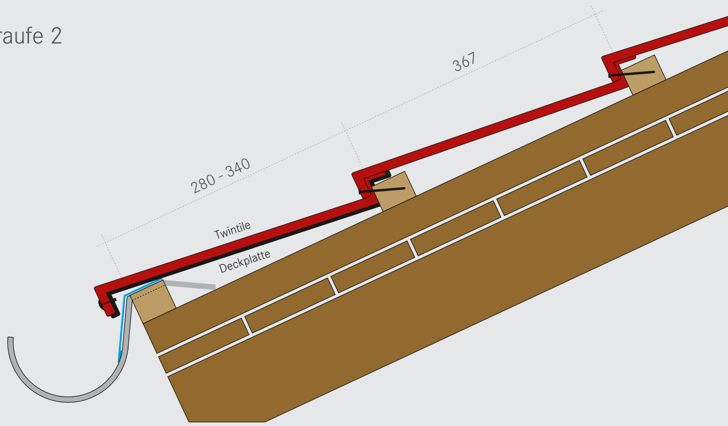
TRAUFE SAUMSTREIFEN AUS DECKPLATTE
